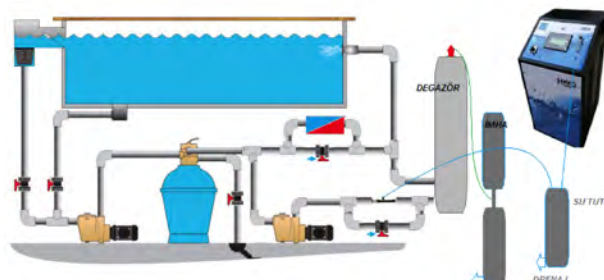
Dozon Maxi Degazör Montaj Şeması Dozon Maxi Degastor Assembly Diagram
